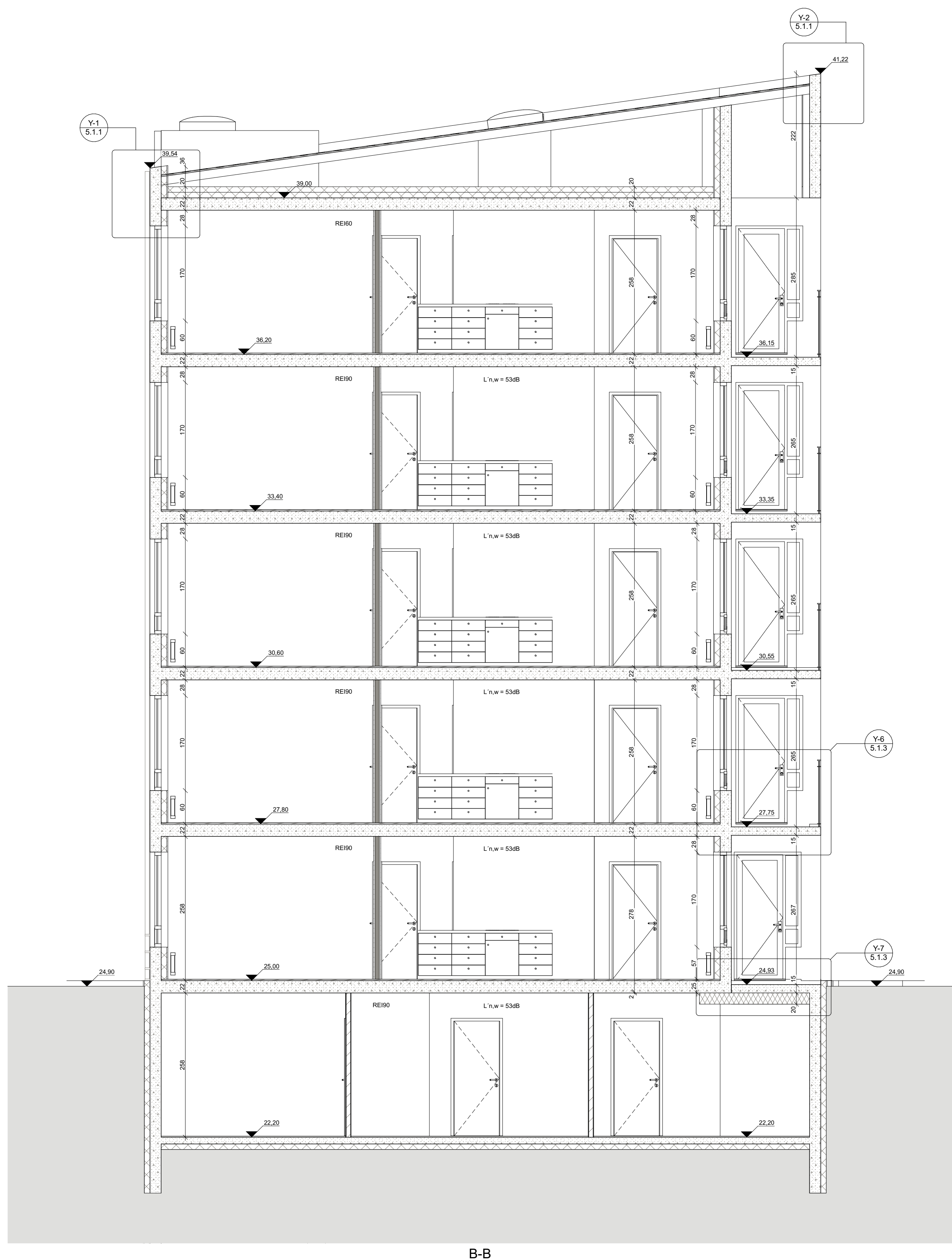
B-B
